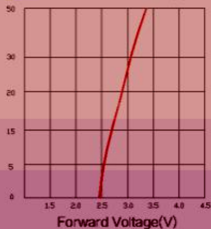
正向电压与正向电流特性曲线
